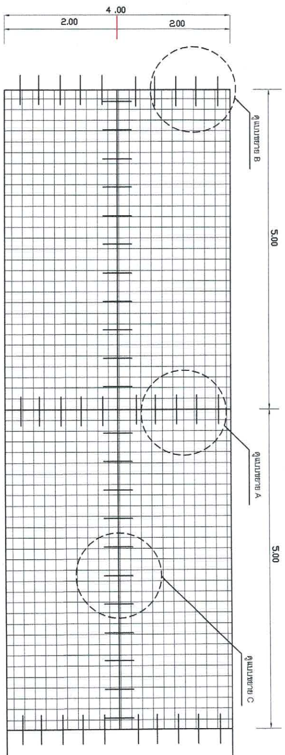
แบบแสดงการก่อสร้างถนนคสล.
